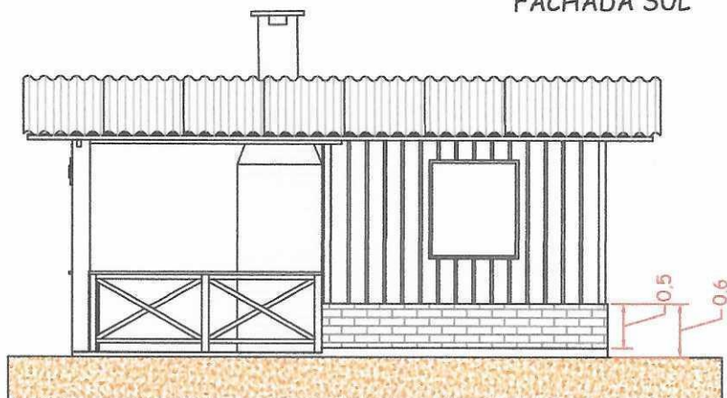
FACHADA LESTE
