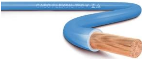
42 - FIO 4,0 mm 2 ISOLAÇÃO 750V
