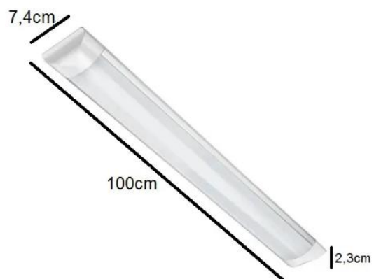
52 - LUMINÁRIA SLIM FIT 36W
